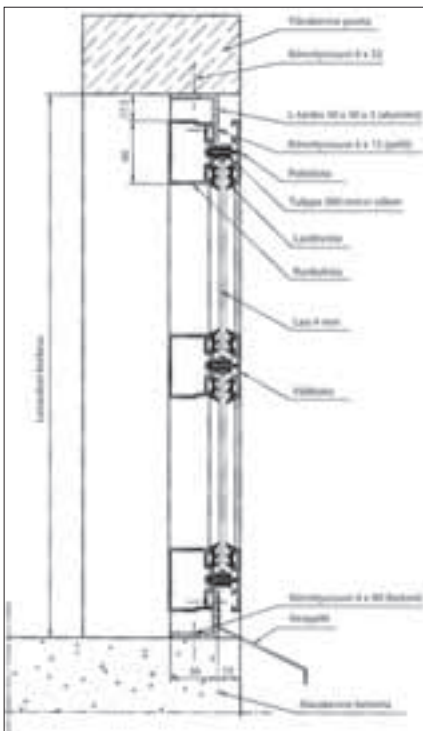
Kiinteän 1-lasisen seinän asennus L-listalla
